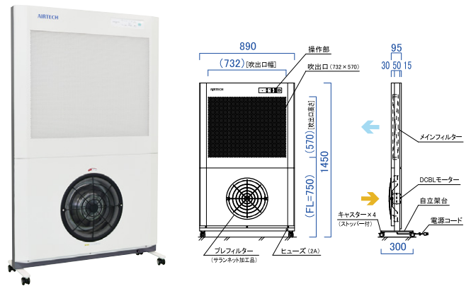
ACP-897BH (クリーン仕様)
