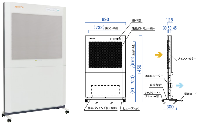
ACP-897CH (汚染除去仕様)
