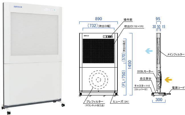
ACP-897AH (クリーン仕様)
